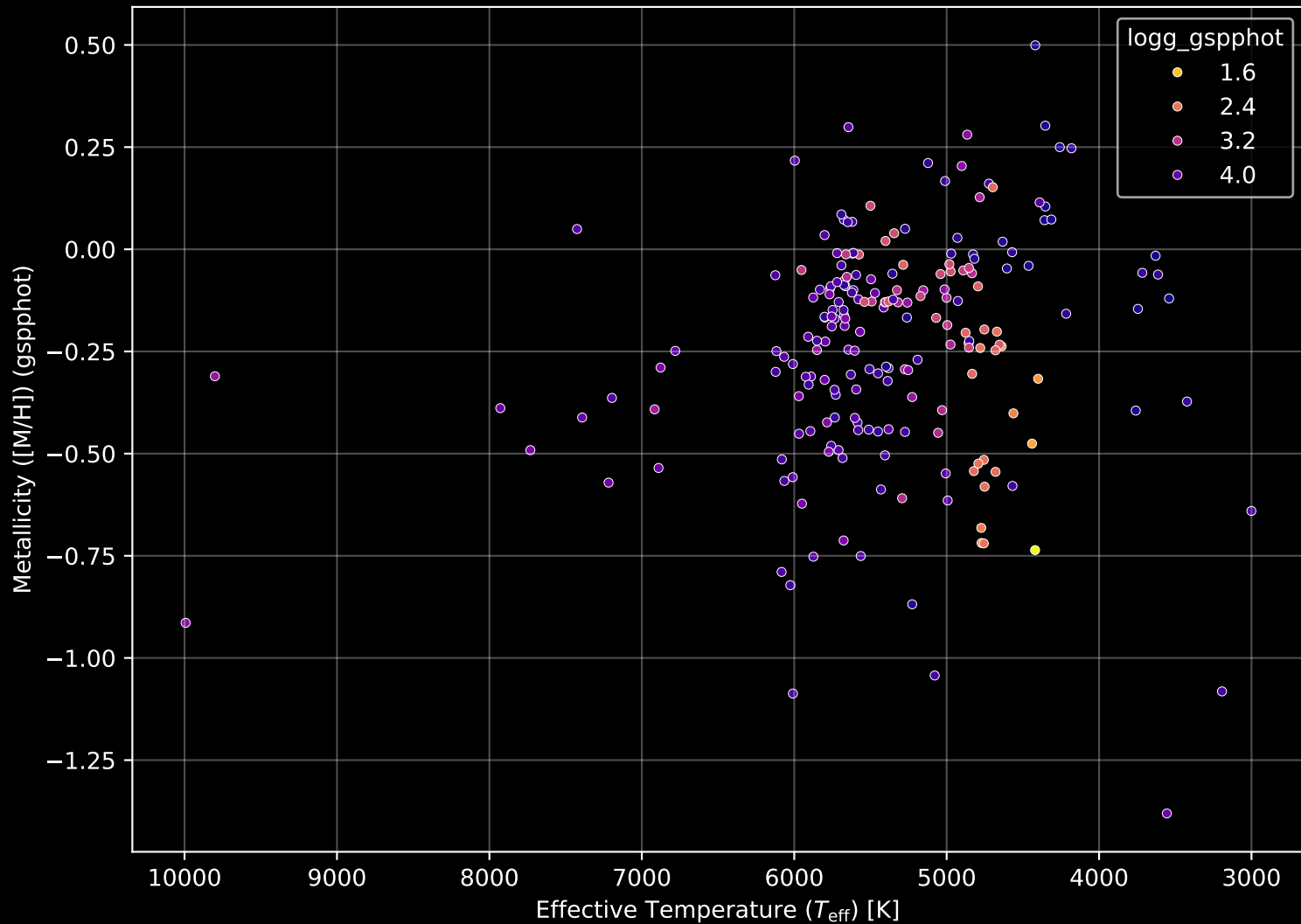
APOGEE DR17 Field: [184+31] Stellar Population Parameters (n= 207)
